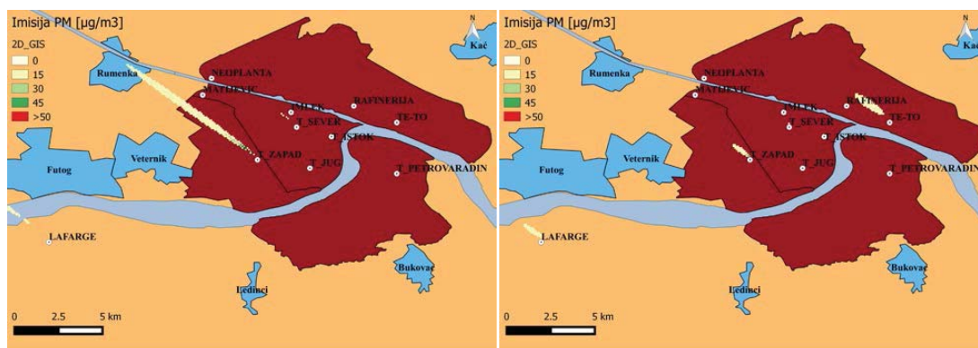
Слика 4.27. Нивои PM за случај југоисточног ветра при стабилној атмосфери (лево) и нестабилној атмосфери (десно)
