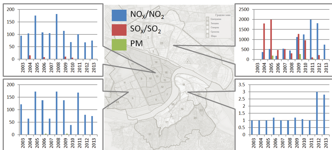
Слика 4.11. Укупна количина емисије \text{NO}_x/\text{NO}_2 , \text{SO}_x/\text{SO}_2 и прашкастих материја (t/години) из стационарних извора, по зонама унутар Агломерације, по годинама. Зоне у којима није било емисије нису приказане
