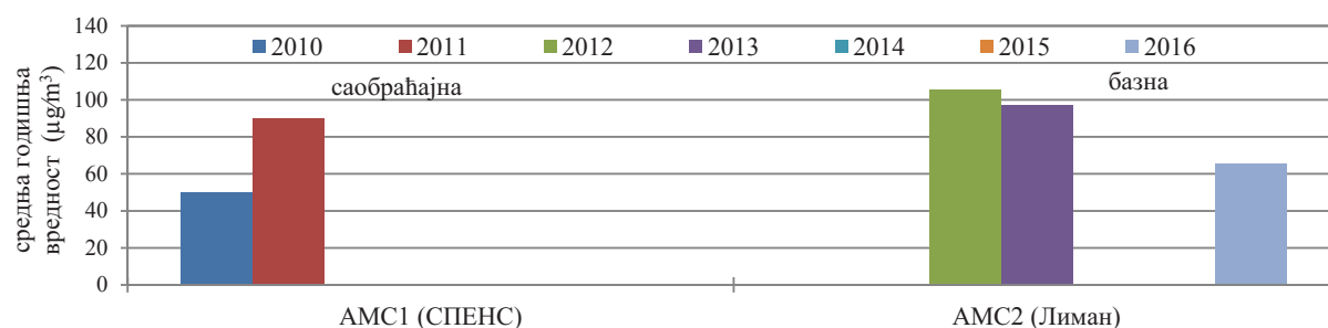
Слика 3.6. Просечне концентрације \text{CO} ( \text{mg}/\text{m}^3 ) у летњој половини године на аутоматским мерним станицама за период 2010-2016. година
