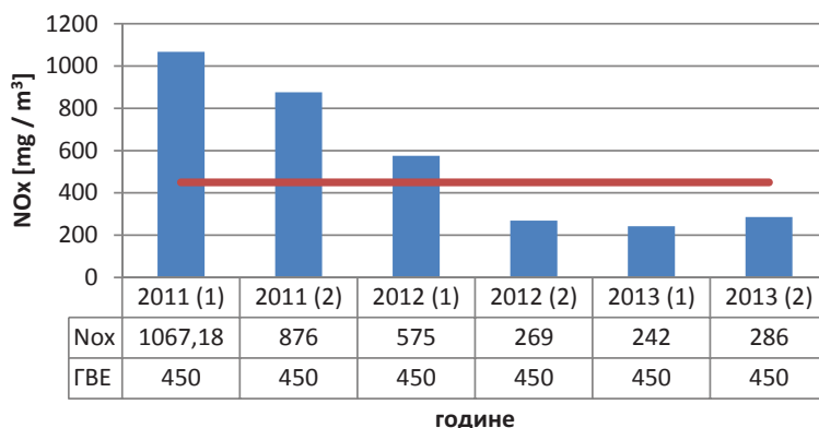
Слика 4.9. Количина емисије NOx/NO 2 у mg/m 3 за НИС – рафинерија „Нови Сад“, по годинама. Број у загради означава редни број мерења у наведеној години, док је црвена линија ГВЕ граница прописана тада важећом Уредбом о граничним вредностима емисија загађујућих материја у ваздух
