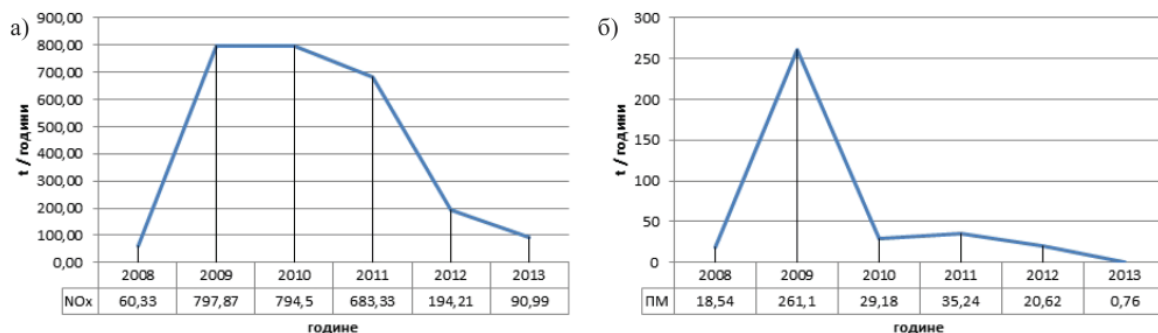
Слика 4.10. Укупна количина емисије (а) \text{NO}_x/\text{NO}_2 и (б) прашкастих материја за НИС – рафинерију „Нови Сад“, према подацима СЕПА по годинама
