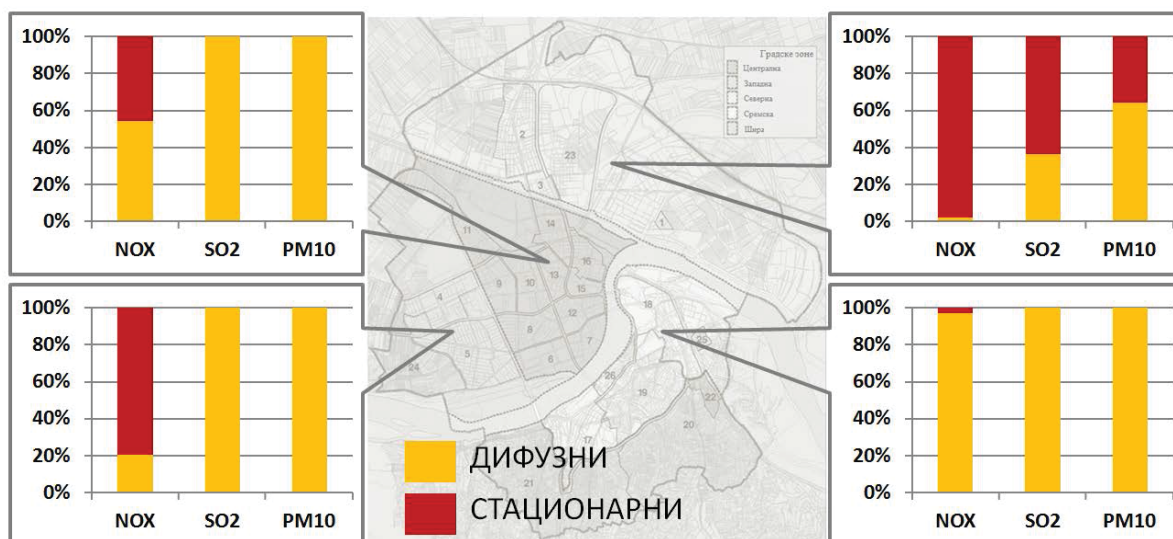
Слика 4.16. Допринос дифузних (индивидуална ложишта) и стационарних (индустрија, енергетика, даљинско грејање) извора емисије укупној емисији по зонама Агломерације
