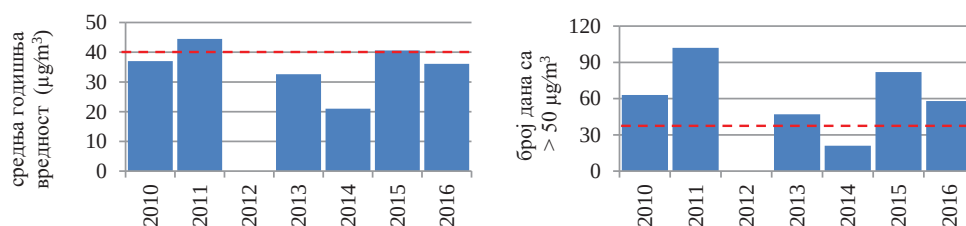
Слика 3.3. Број дана са прекорачењем ГВ и просечне годишње концентрације PM_{10} ( \mu g/m^3 ) на аутоматској саобраћајној мерној станици АМС1 (Дневник/СПЕНС) за период 2010-2016. година
