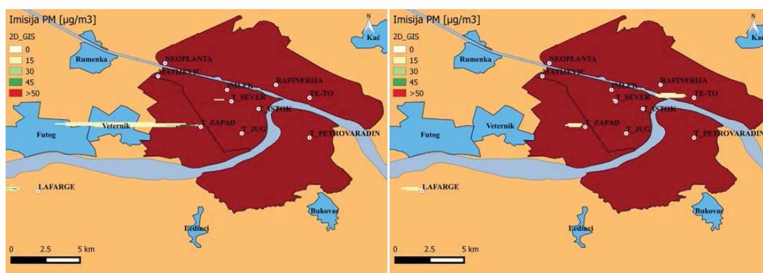
Слика 4.25. Нивои PM за случај источног ветра при стабилној атмосфери (лево) и нестабилној атмосфери (десно)
