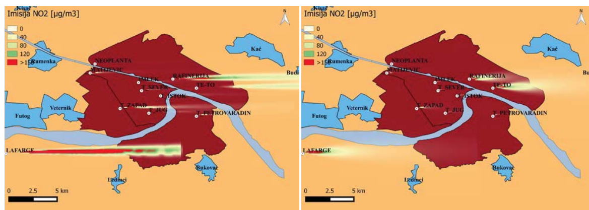
Слика 4.20.. Нивои \text{NO}_2 за случај западног ветра при стабилној атмосфери (лево) и нестабилној атмосфери (десно)
