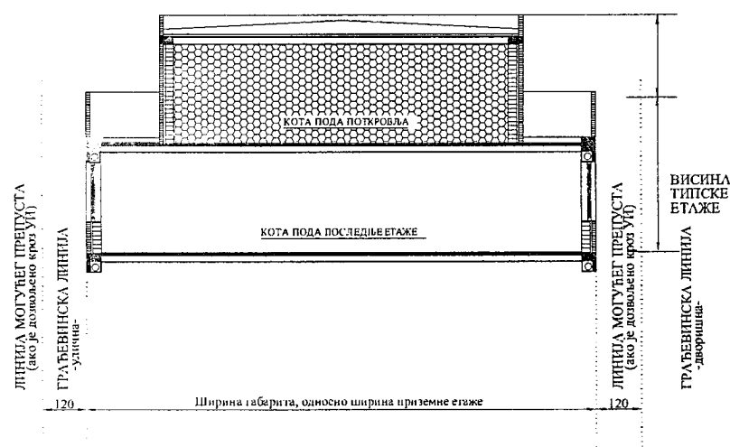
Начин формирања равнoг крова са кровном етажом-карактеристичан пресек
