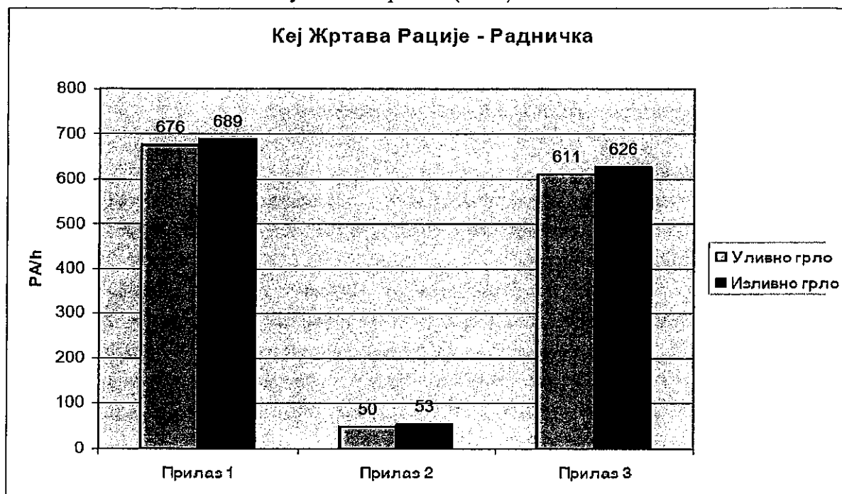
Слика 4. Величине токова по уливним грлима (РА/х)
