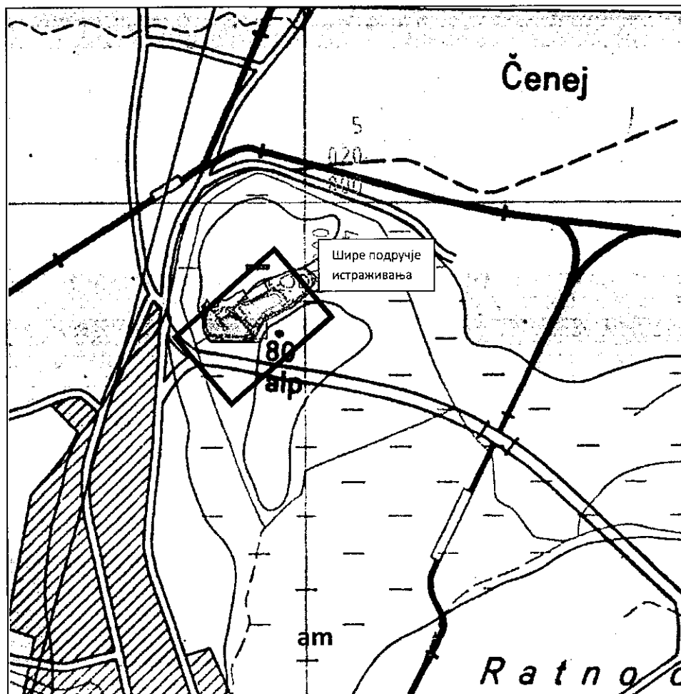
Слика 2. Прегледна геолошка карта ширег истражног подручја (извор: ОФГ Лист Нови Сад L 34-100, 1:100 000)
