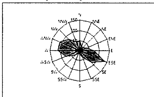
Слика 3. Ружа ветрова за климатолошку станицу „Римски Шанчеви“ (просек 1981. – 2010. године)
