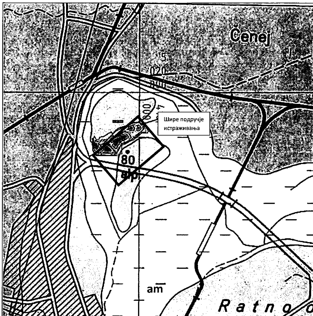
Слика 1: Прегледна геолошка карта ширег истражног подручја (извор: ОФГ Лист Нови Сад L 34-100, 1:100 000)
