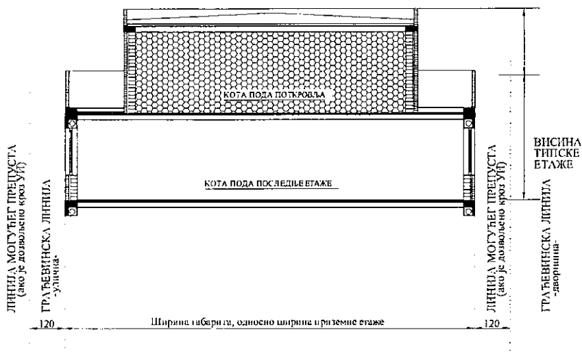
Слика: Начин формирања равног крова са кровном етажом – карактеристичан пресек
