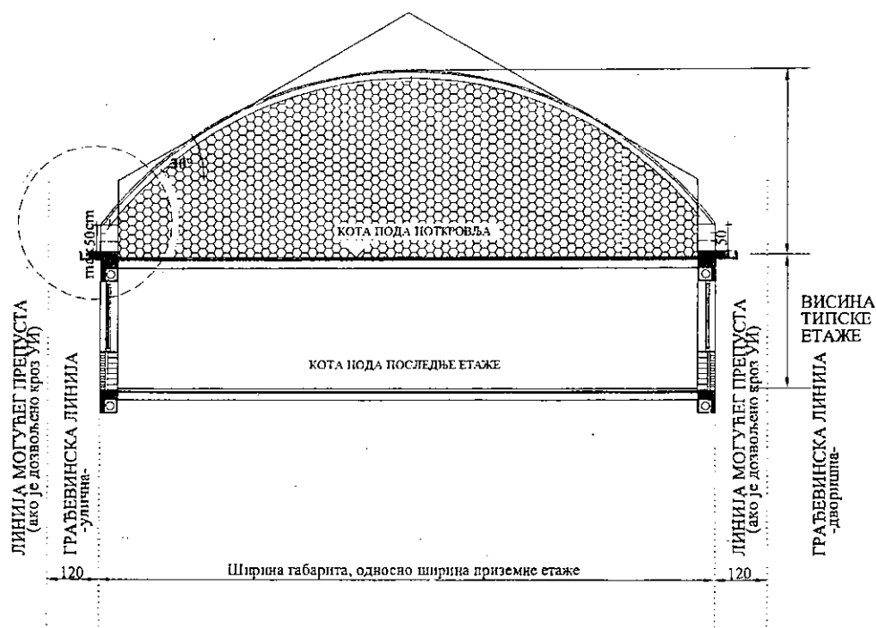
Скица: Начин формирања лучних кровова – карактеристични пресек.
