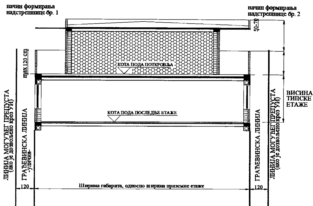
Слика број 4: Начин формирања равног крова са кровном етажом – карактеристичан пресек
