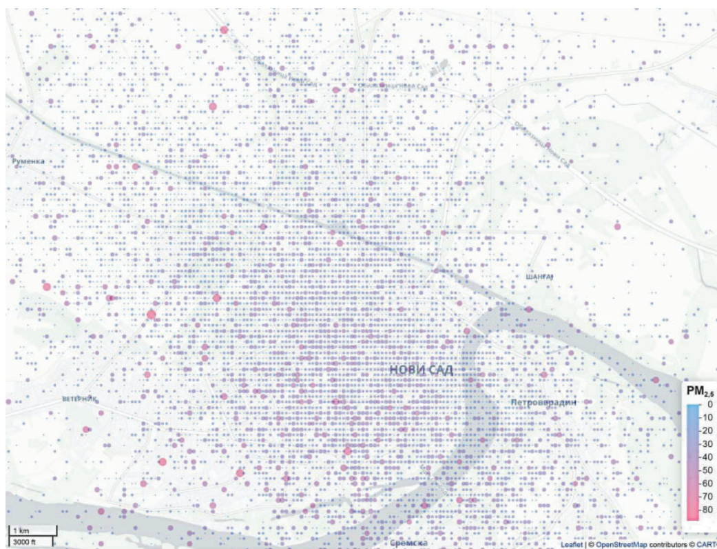
Слика 70. Распдела извора емисије PM_{2.5} на територији Новог Сада и суседних општина у периоду од 2018. до 2020. године
