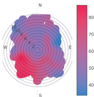
Слика 43. Зависност концентрација O_3 [ \mu\text{g m}^{-3} ] од правца и брзине ветра на мерном месту Лиман у Новом Саду за период од 2018. до 2020. године
