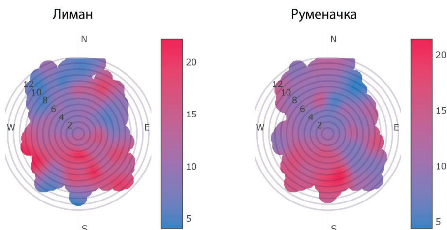
Слика 42. Зависност концентрација SO_2 [ \mu\text{g m}^{-3} ] од правца и брзине ветра у Новом Саду за период од 2018. до 2020. године
