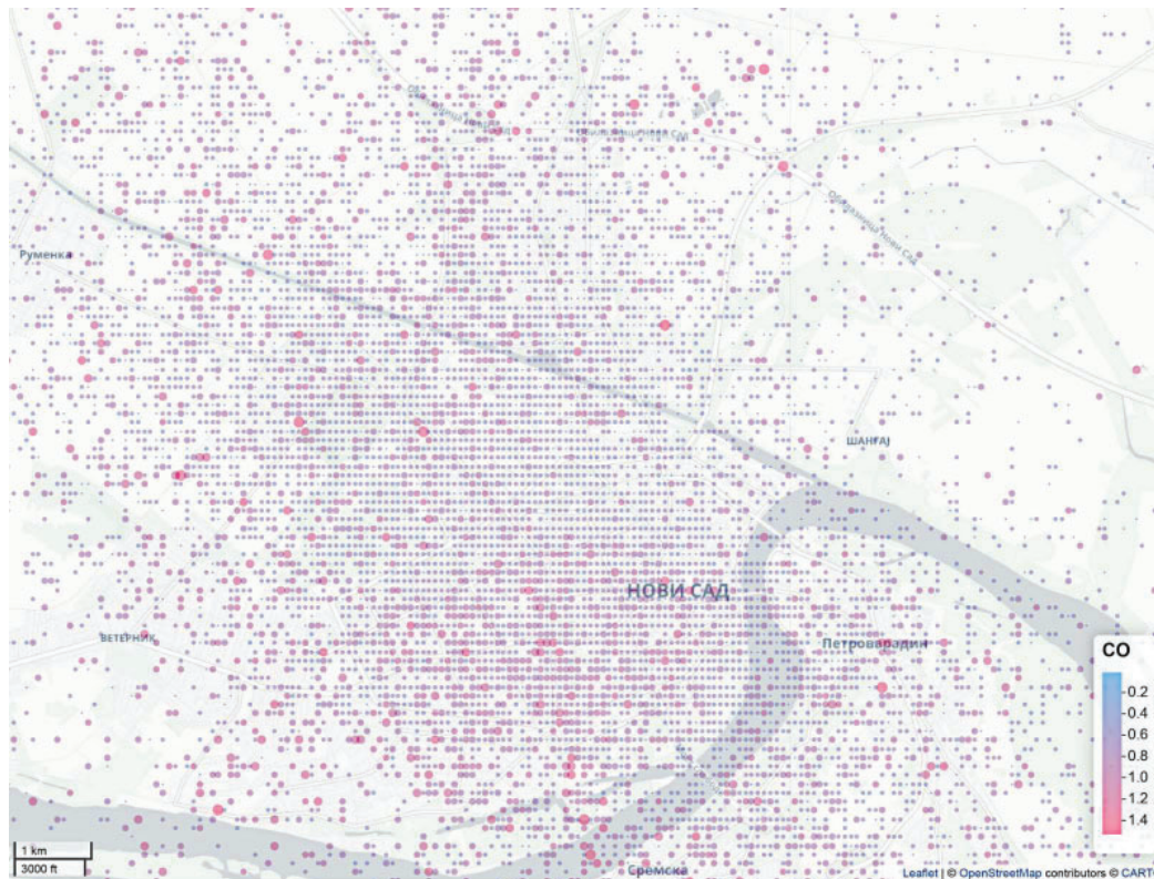
Слика 71. Распдела извора емисије CO на територији Новог Сада и суседних општина у периоду од 2018. до 2020. године
