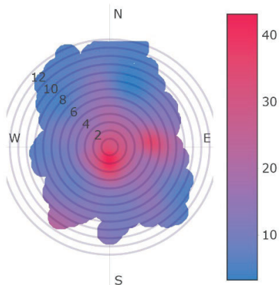
Слика 23. Зависност концентрација PM_{2.5} [ \mu\text{g m}^{-3} ] од правца и брзине ветра на мерном месту Руменачка у Новом Саду за период од 2018. до 2020. године
