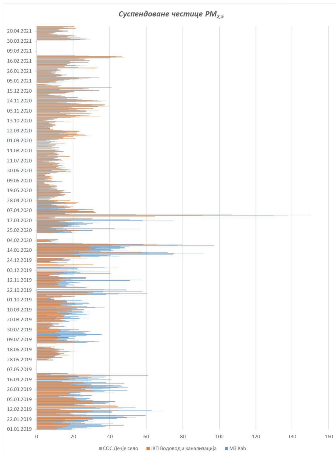
Слика 29. Приказ максималне и минималне концентрације суспендованих честица PM_{2,5} ( \mu g/m^3 ) на мерним станицама Месна заједница „Каћ“, ЈКП „Водовод и канализација“ ППДВ и СОС Дечје село „Др Милорад Павловић“ за период од 2019. до 2020. године
