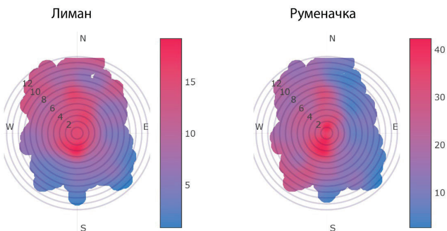
Слика 41. Зависност концентрација NO 2 [ \mu\text{g m}^{-3} ] од правца и брзине ветра у Новом Саду за период од 2018. до 2020. године
