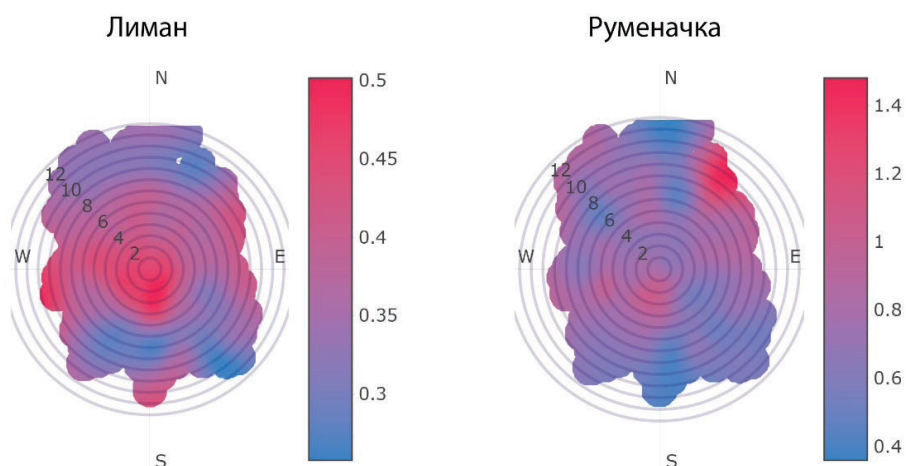
Слика 40. Зависност концентрација CO [ \text{mg m}^{-3} ] од правца и брзине ветра у Новом Саду за период од 2018. до 2020. године
