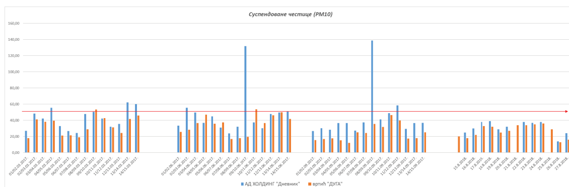
Слика 24. Дневне варијације концентрација суспендованих честица PM_{10} у ваздуху на мерним местима АД Холдинг "Дневник" и вртић "Дуга" током периода 2017 -2018. година
