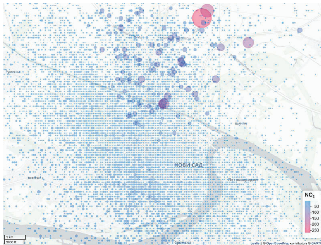
Слика 73. Распдела извора емисије NO 2 на територији Новог Сада и суседних општина у периоду од 2018. до 2020. године
