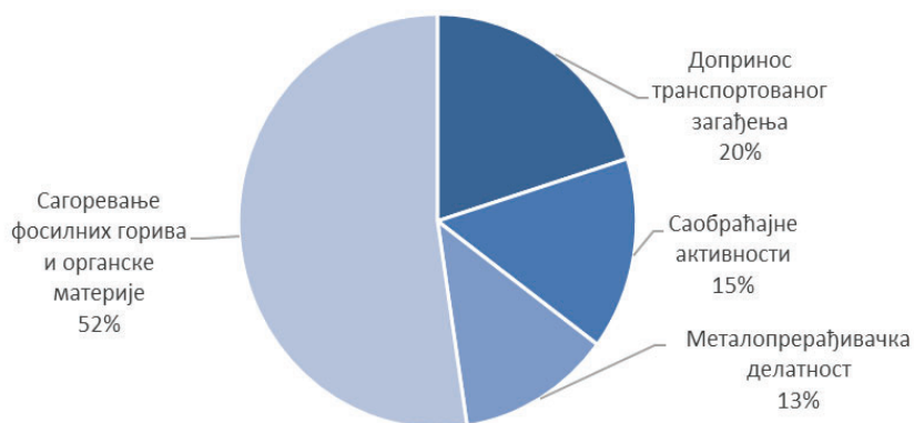
Слика 105. Удео доминантних извора емисије на мерном месту Неопланта ад Нови Сад током 2021. године
