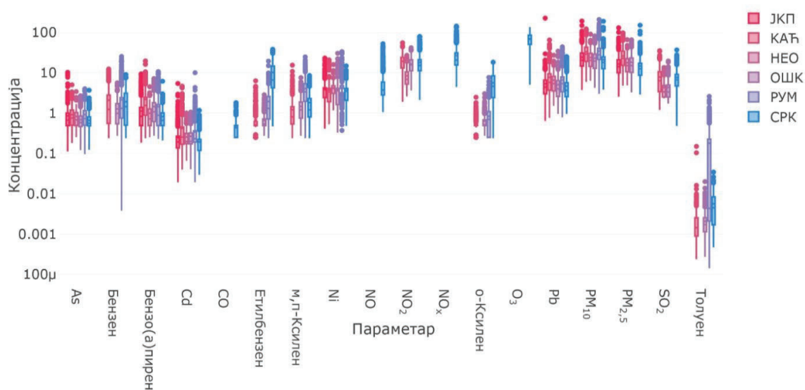
Слика 86. Дескриптивна статистика дневних концентрација загађујућих материја на мерним местима у Новом Саду за период од 2019. до августа 2021. године
