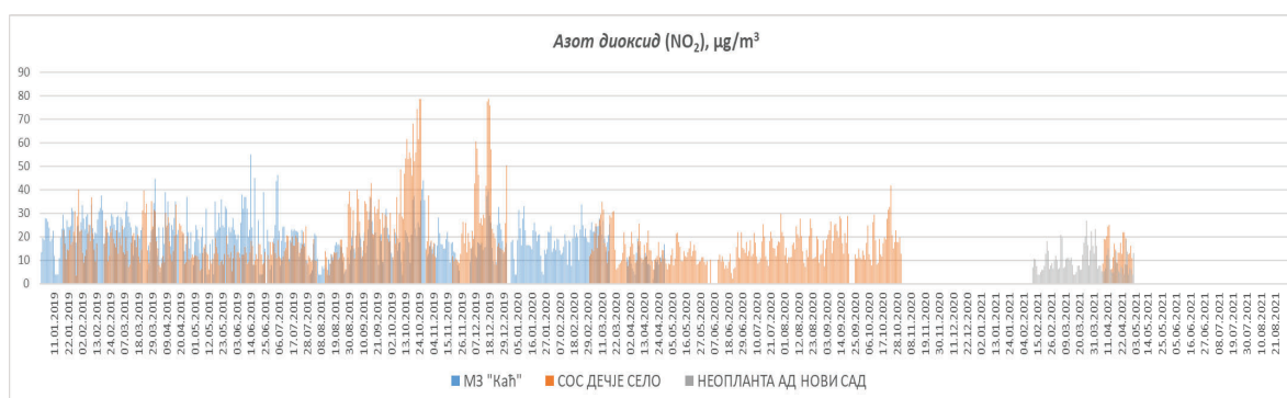
Слика 23. Дневне варијације концентрација \text{NO}_2 на мерном месту Месна заједница "Кањ", СОС ДЕЧЈЕ СЕЛО „Др Милорад Павловић“ и НЕОПЛАНТА АД Нови Сад током периода 2019-2021 ( \mu\text{g}/\text{m}^3 )
