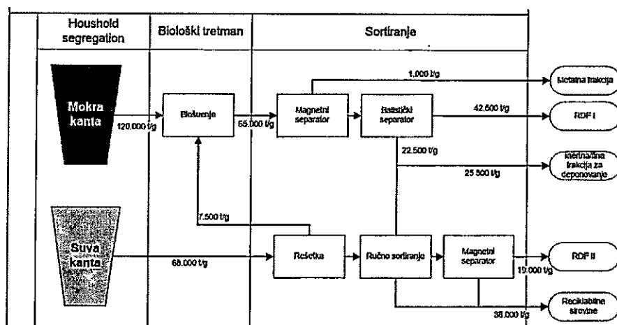
Слика 5.8 Општи масени биланс MBT постројења на бази процеса био-сушења
