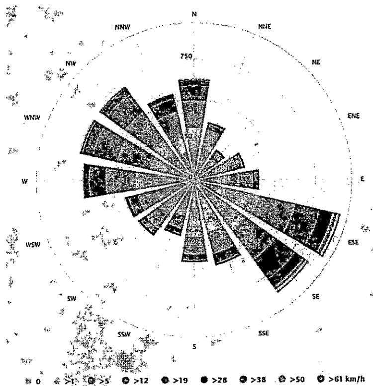
Слика 2.3 Ружа ветрова за Град
