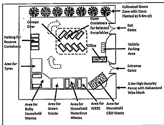
Слика 5.9 Општи изглед рециклажног дворишта
