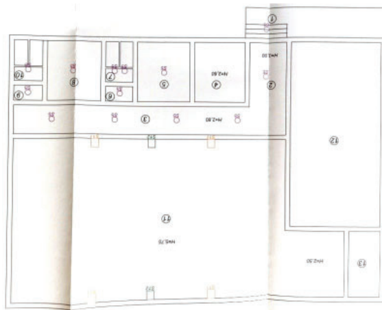
Слика 5. Нацрт објекта - фискултурна сала
