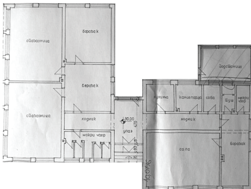
Слика 5. Нацрт објекта са означеним просторијама
