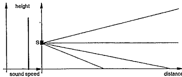
Слика 29. Приказ хомогених услова простирања звука
