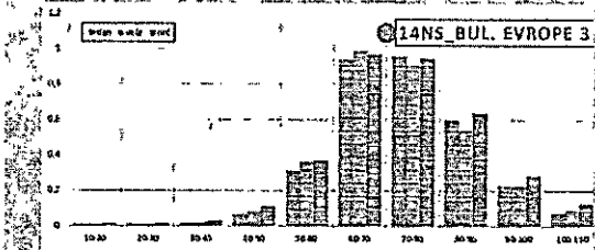
Дијаграм 13. Подаци о броју и брзини кретања возила за дан, вече и ноћ за бројача 14НС Бул. Европе 3
