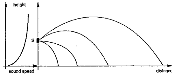
Слика 28. Приказ рефракције звука
