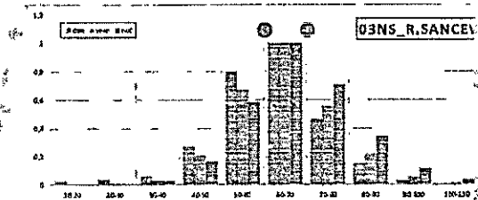
Дијаграм 3. Подаци о броју и брзини кретања возила за дан, вече и ноћ за бројача 03НС Р.Шанчеви
