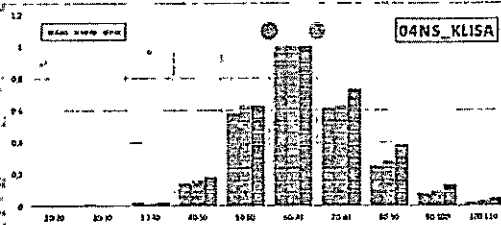
Дијаграм 4. Подаци о броју и брзини кретања возила за дан, вече и ноћ за бројача 04НС Клица
