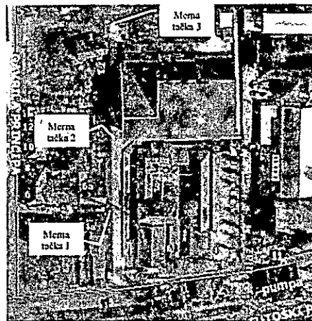
Слика 20. Позиције мерних места и резултати мерења за објекат ТО „Запад“
