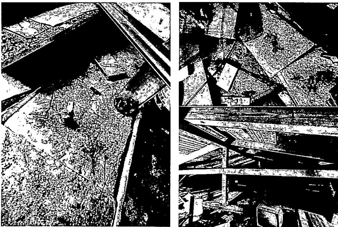
Слика 7 - Изглед међуспратне конструкције испод негрејаног простора
