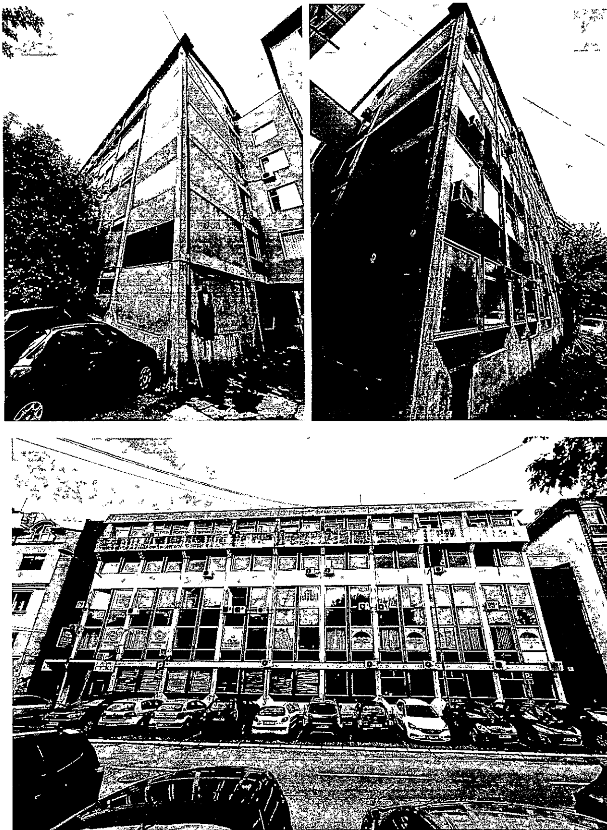
Слика 5 - Изглед спољних зидова објекта
