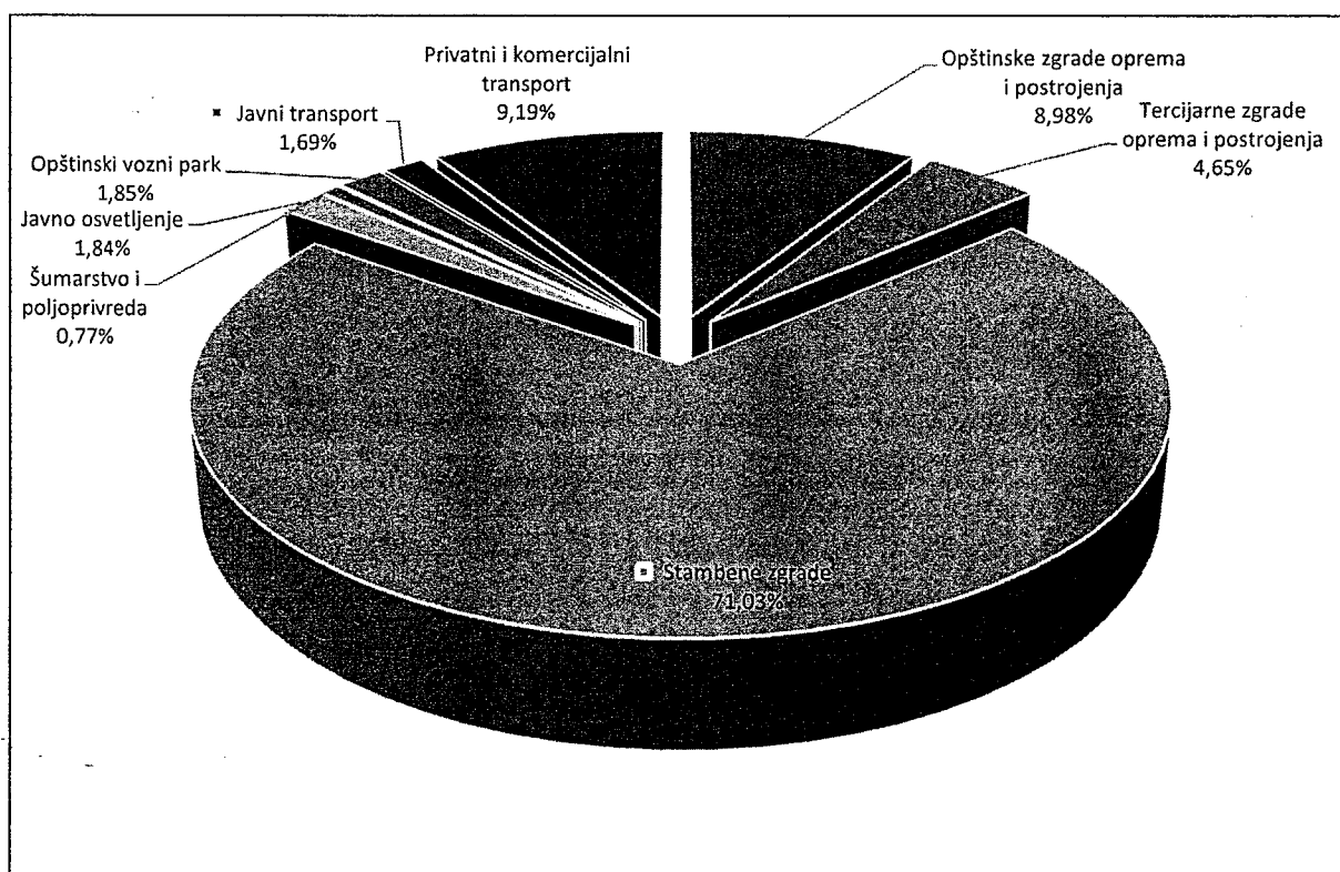
Дијаграм 15. Процентуална емисија CO 2 по секторима потрошње
