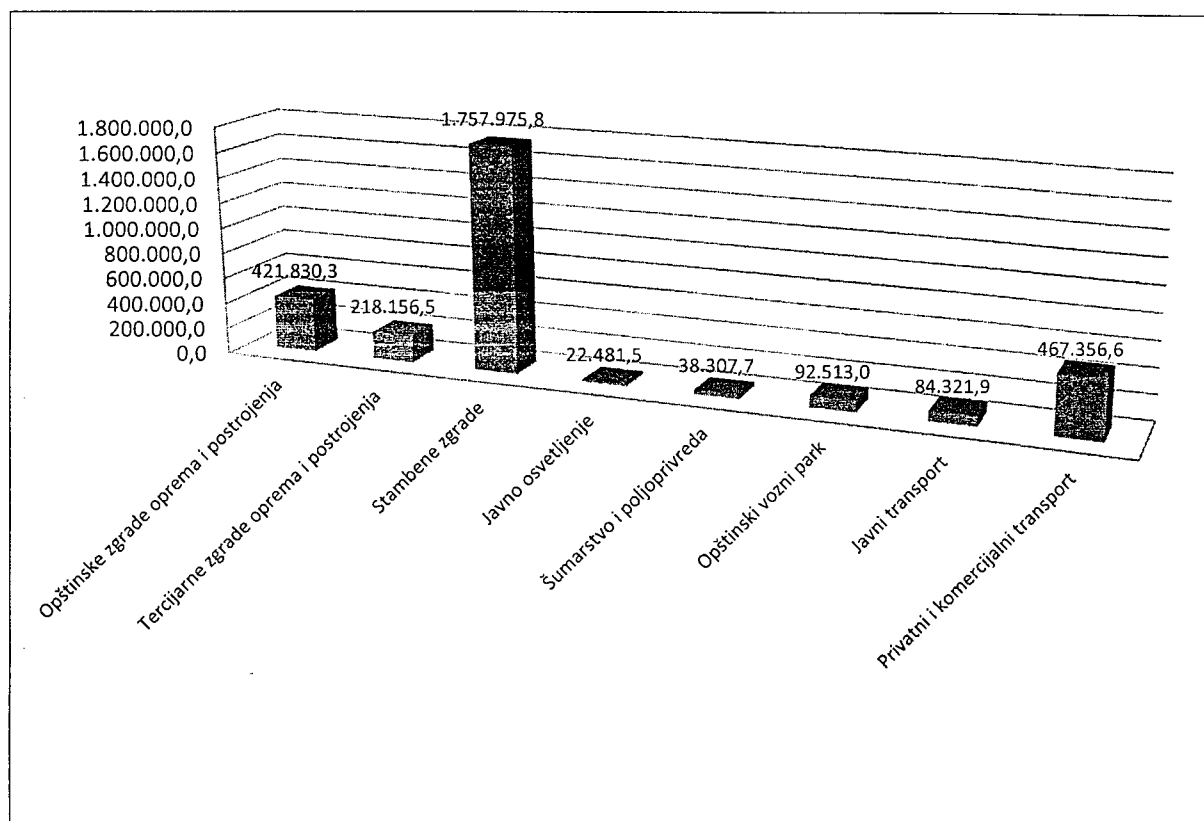
Дијаграм 10. Потрошња финалне енергије по секторима
