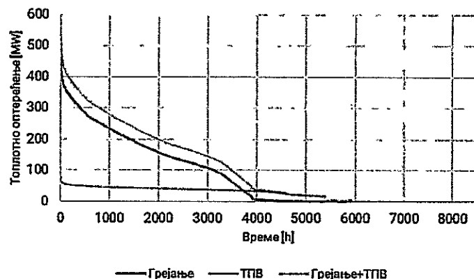
Слика 4.3 - Типична крива трајања оптерећења за ЈКП "Новосадска топлана" (Грејање и ТПВ)
