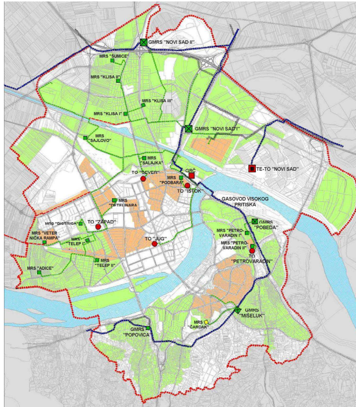
Слика 4.13 – Приказ гасоводне мреже Града Новог Сада
